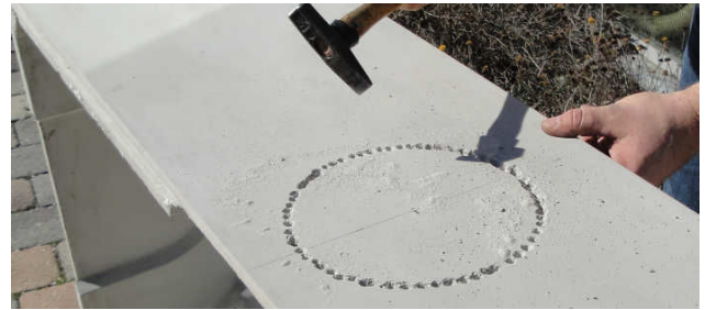
Bild 5: Skära urtag med en bormaskin
