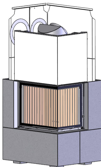
Bild 7: Installera strålningsplåtarna (om önskade)
