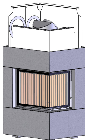
Bild 8: Sätt på den tredje ringen
